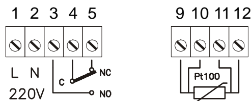
Rys. 3. Podłączenia do regulatora współpracującego z czujnikiem Pt100
