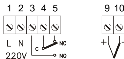
Rys. 2. Podłączenia do regulatora współpracującego z czujnikiem termoparowym
