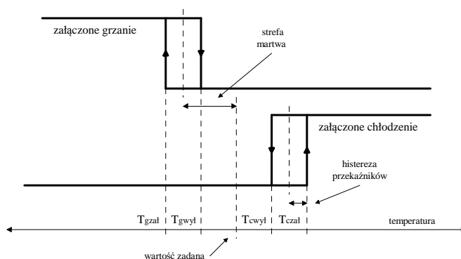
Rys. A. Algorytm pracy regulatora ST-51
