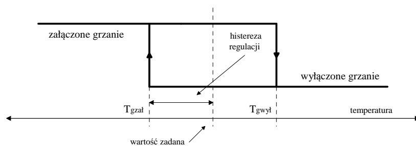
Rys. 2. Algorytm pracy regulatora ST-54
