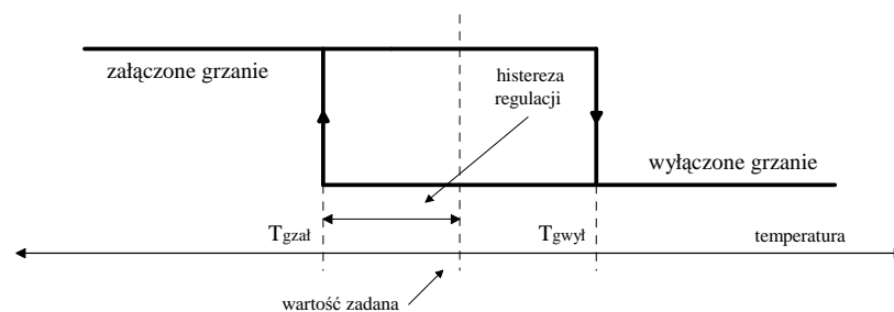
Rys. 2. Algorytm pracy regulatora ST-701
